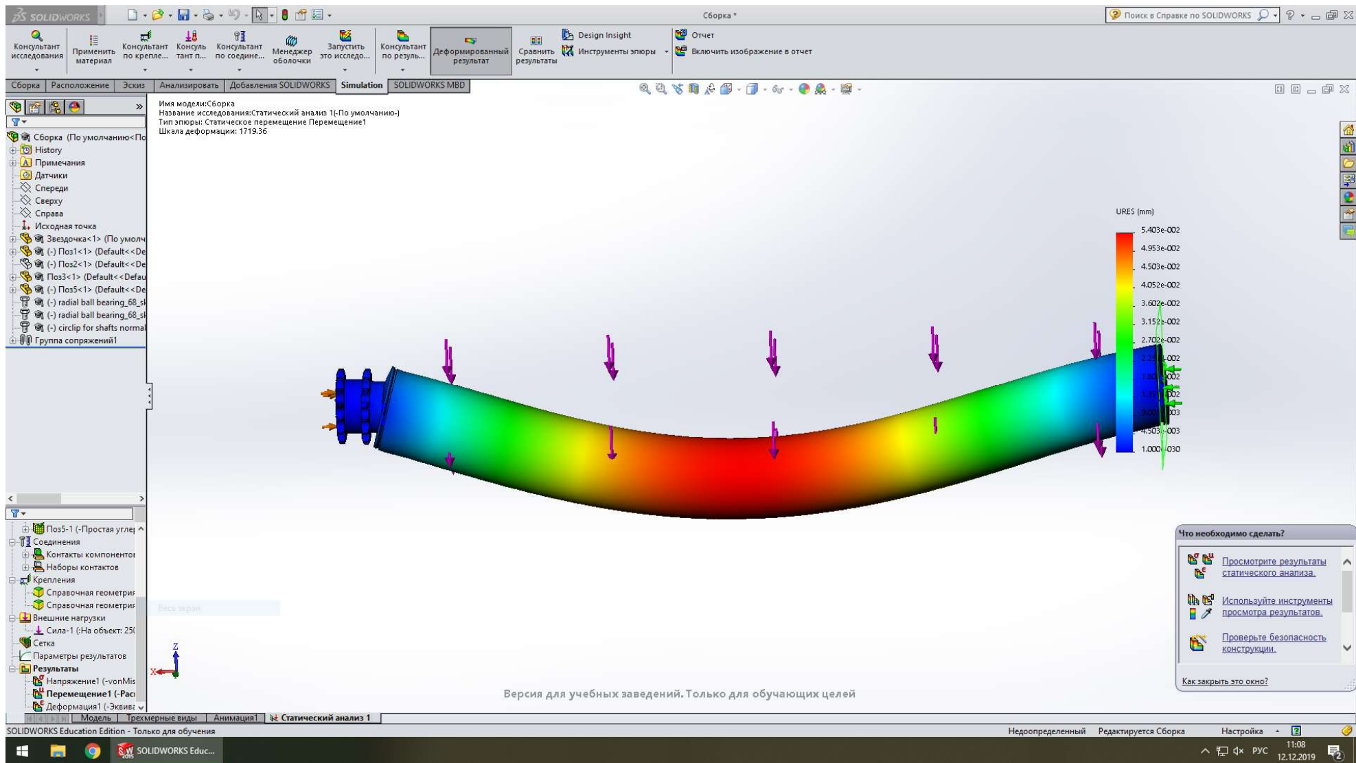
Рисунок 2 – Перемещения, возникающие в ролике при нагрузке
