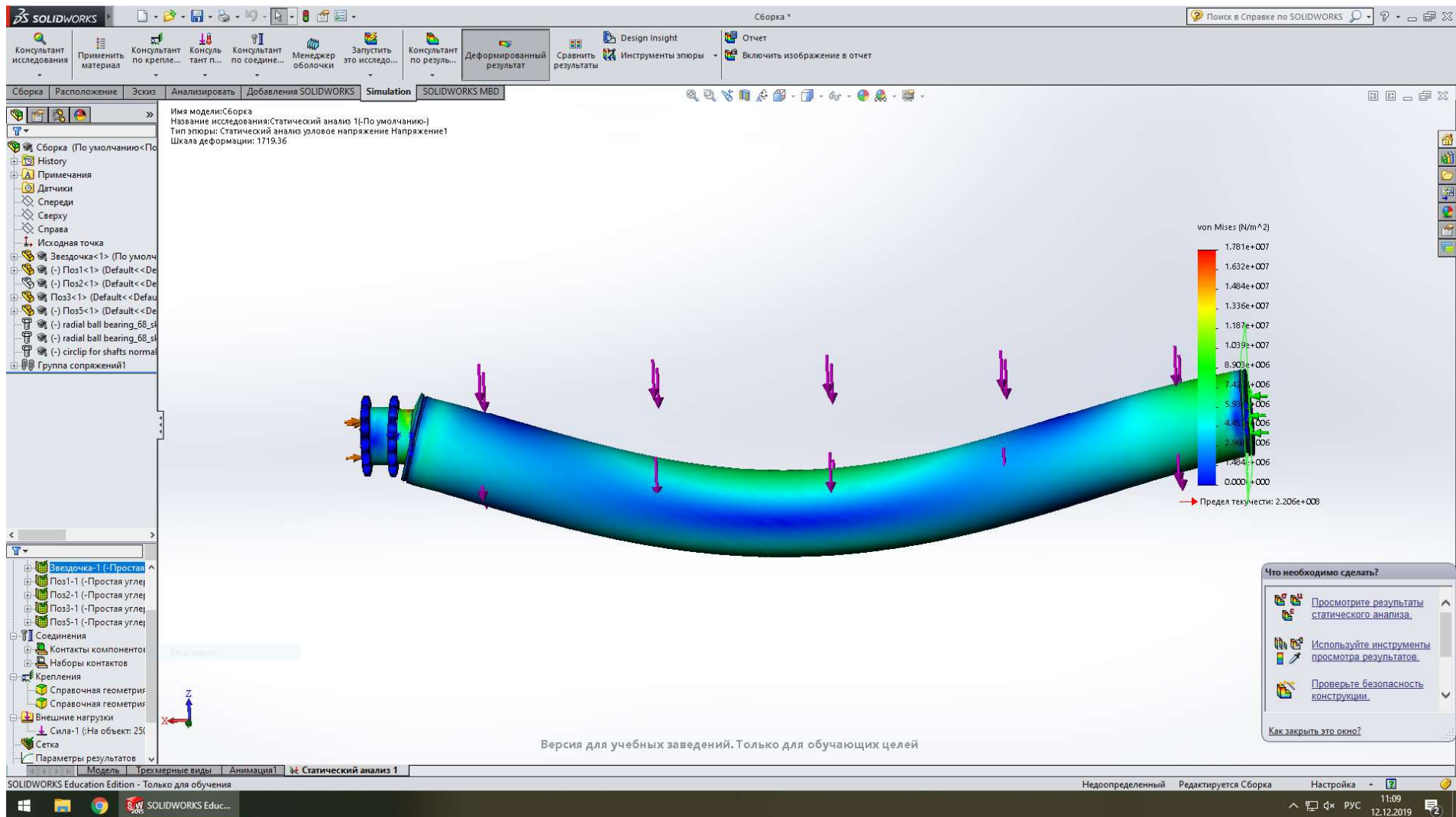
Рисунок 1- Напряжения, возникающие в ролике при нагрузке
