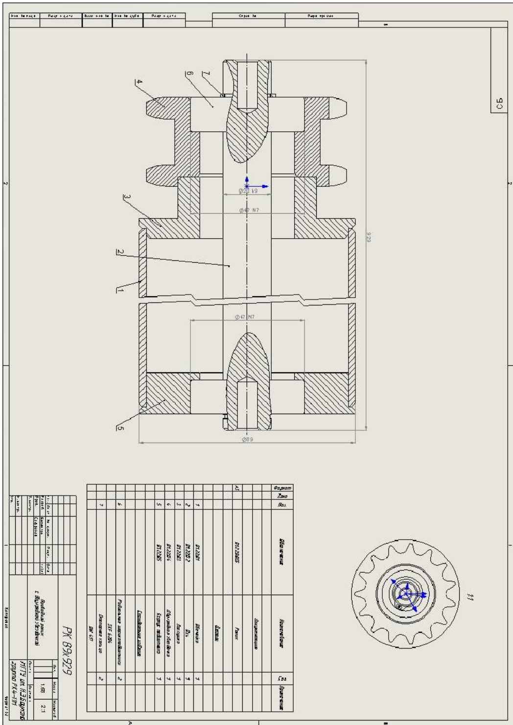
Рисунок 1. Сборочный чертеж приводного ролика
